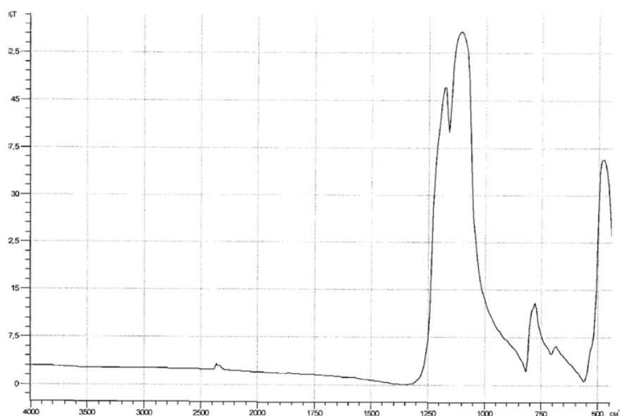
Рис. 6. Типичный ИК-спектр МНПВО жильного кварца Тасеевского месторождения малоглубинной золото-серебряно-кварцевой формации
