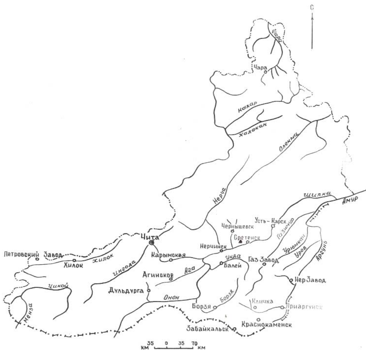
Местонахождение пономарий в юрских отложениях пади Зергун (черный треугольник)
