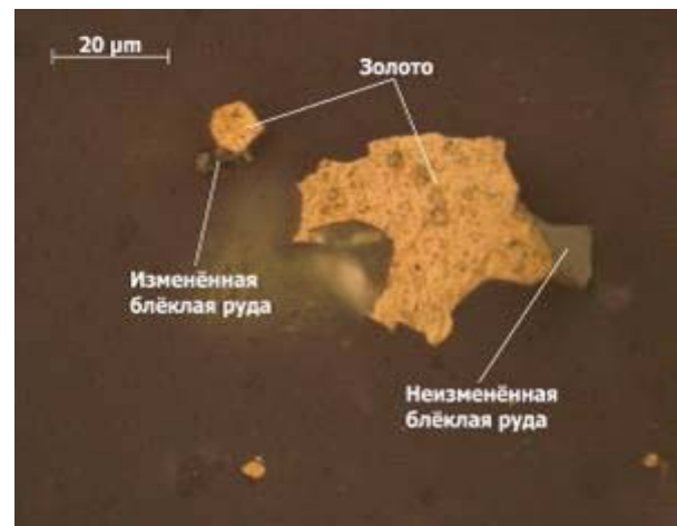
Рис. 4. Формы и размеры выделений золота и блеклой руды в микрозернистом кварце Тасеевского месторождения. Обр. 398-ю
