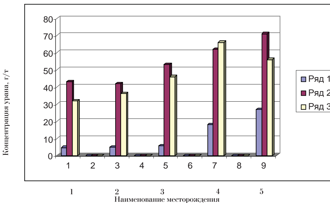
Концентрация урана в углях и продуктах их сжигания на Забайкальских буроугольных месторождениях: 1 – Окино-Ключевское; 2 – Татауровское; 3 – Харанорское; 4 – Уртуйское; 5 – Кутинское; 1 ряд – уголь; 2 ряд – зола; 3 ряд – шлак
