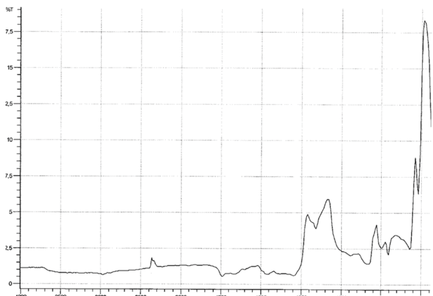
Рис. 5. Типичный ИК-спектр МНПВО жильного кварца Любавинского месторождения среднеглубинной золото-кварцевой формации
