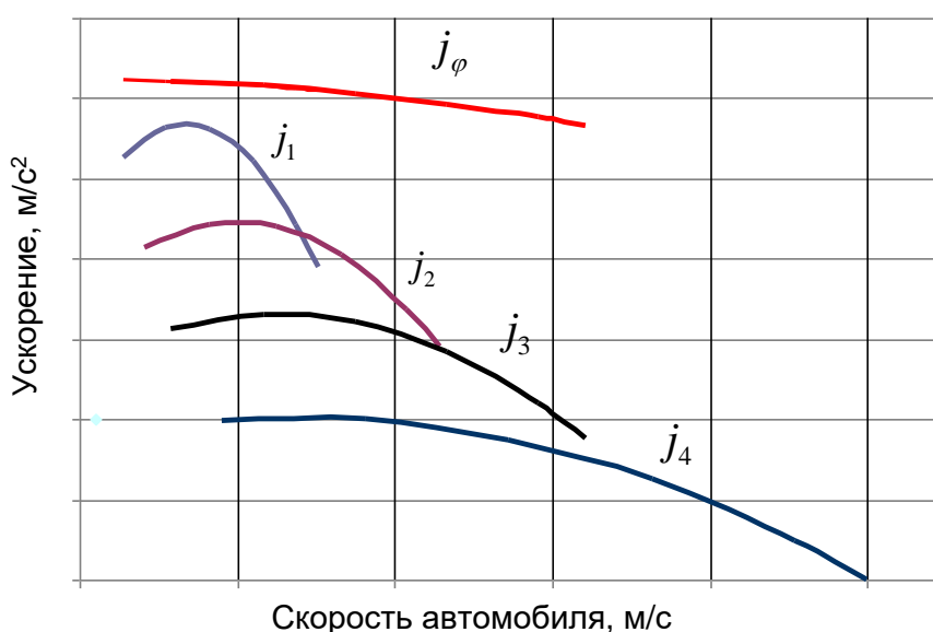
Рис. 6. График ускорений автомобиля при разгоне: j_\phi — ускорение, возможное по условиям сцепления; j_1 - j_4 — ускорения автомобиля на различных передачах по тяговым свойствам
