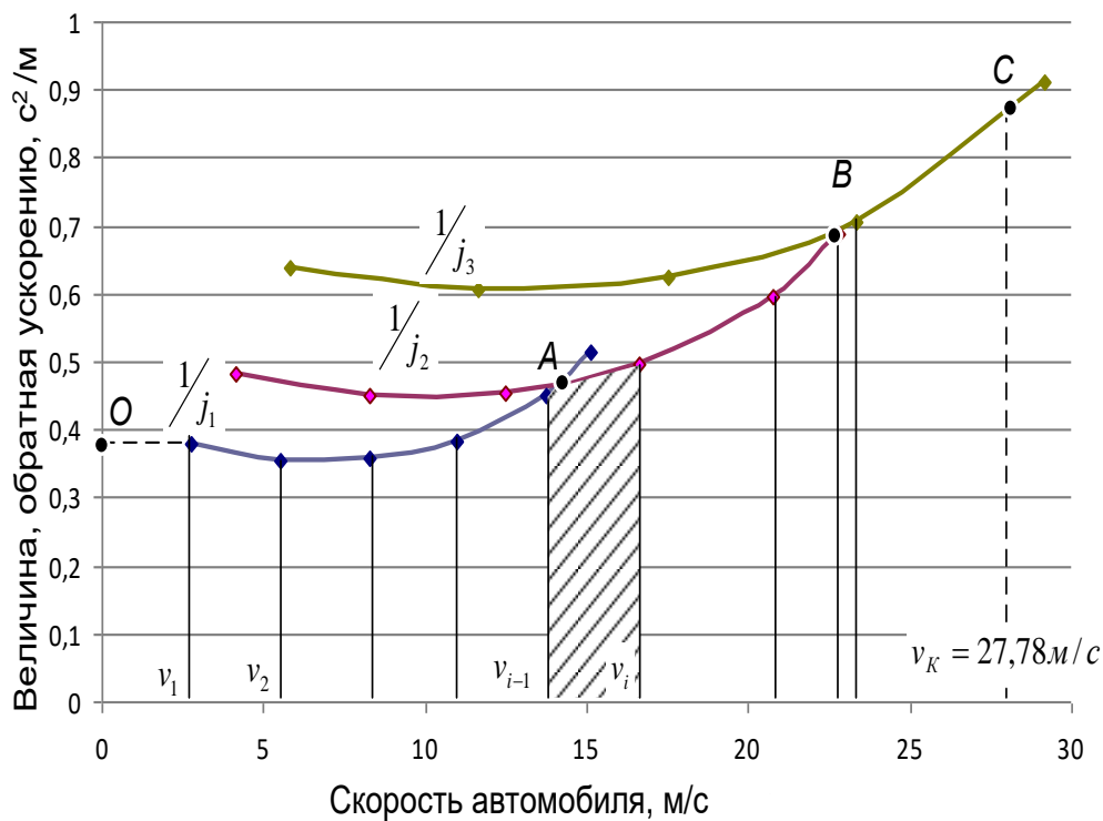
Рис. 7. График величин, обратных ускорениям
