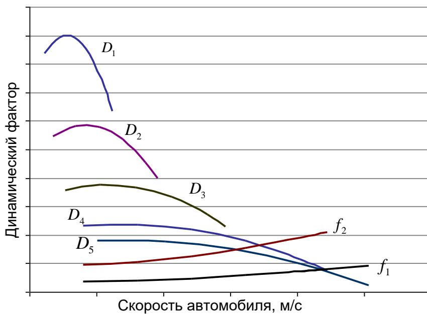
Рис. 5. Динамическая характеристика автомобиля
