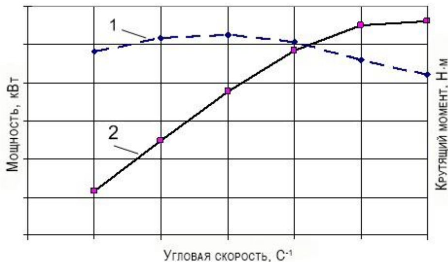
Рис. 1. Внешняя скоростная характеристика двигателя: 1 – крутящий момент; 2 – мощность
