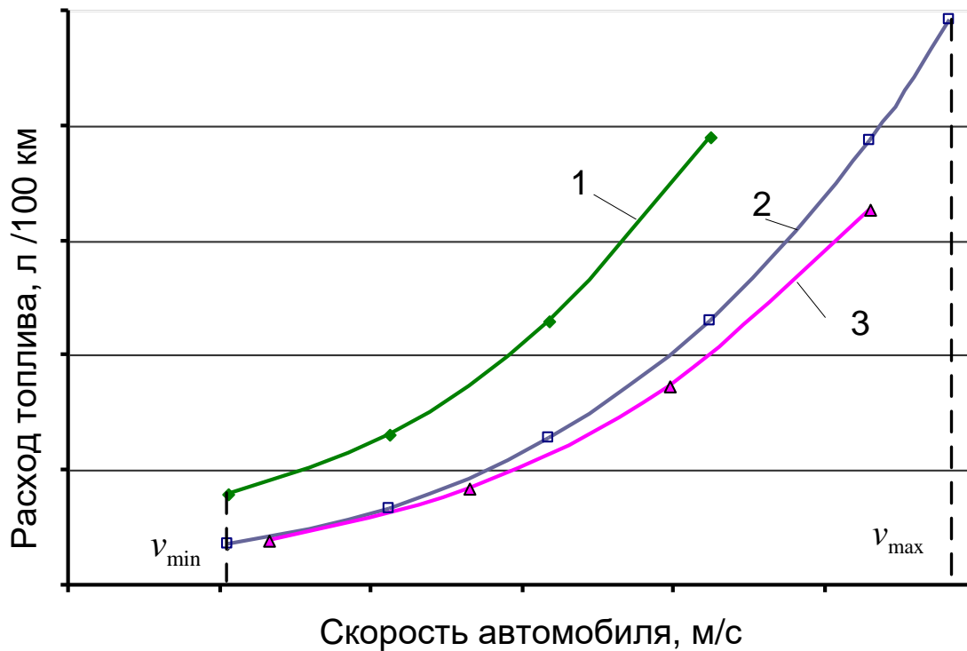
Рис. 10. Топливо-экономическая характеристика автомобиля на прямой (линии 1 и 2) и ускоряющей передаче (линия 3)
