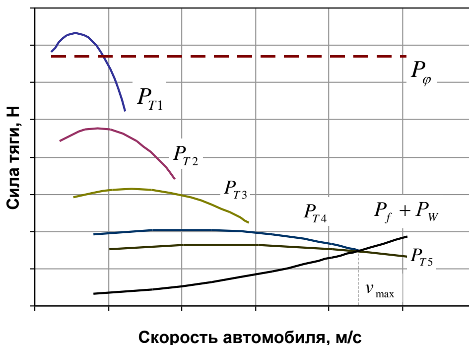
Рис. 3. График тягового баланса автомобиля
