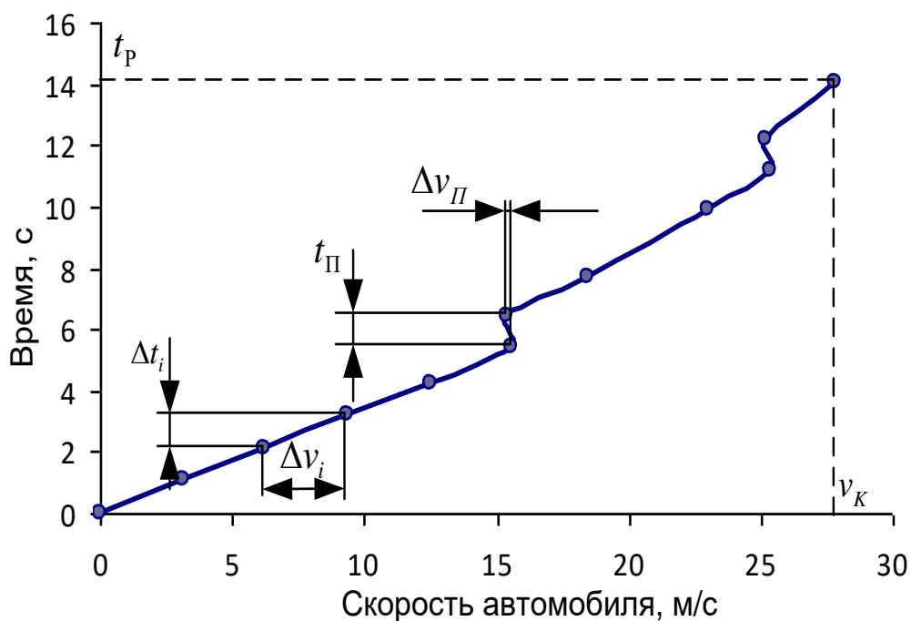
Рис. 8. График времени разгона до контрольной скорости с учетом переключения передач
