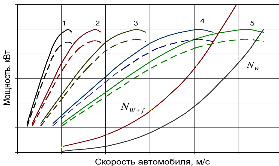
Рис. 4. График мощностного баланса автомобиля: 1, 2, ... 5 – мощностная характеристика на 1-й, 2-й, ... 5-й передачах (сплошные линии – мощность на коленчатом валу двигателя, пунктирные линии – мощность на ведущих колесах); N_w – мощность, необходимая для преодоления силы сопротивления воздуха; N_{w+f} – суммарная мощность, необходимая для преодоления сил сопротивления воздуха и дорожного сопротивления
