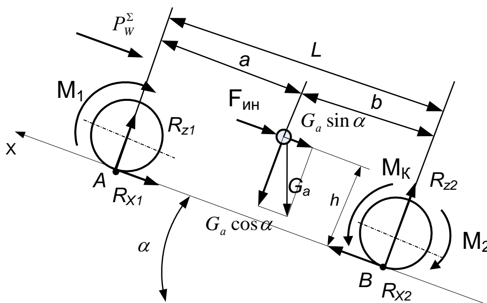
Рис. 2. Силы, действующие на автомобиль в общем случае движения
